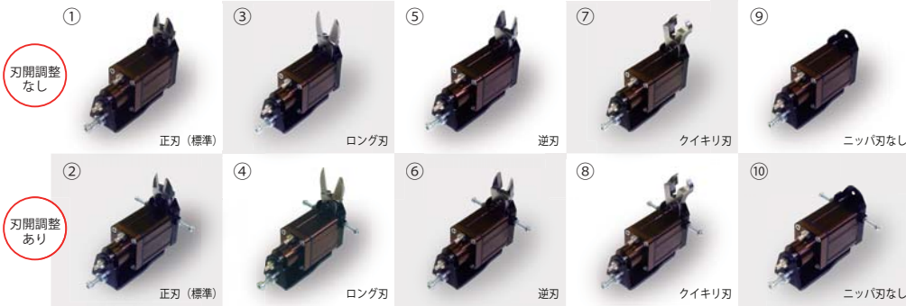
外形寸法図 刃開調整なし
