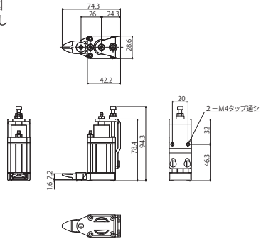
外形寸法図 刃開調整あり
