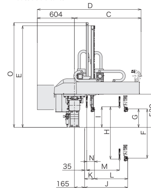
操作側取出仕様 (mm)
