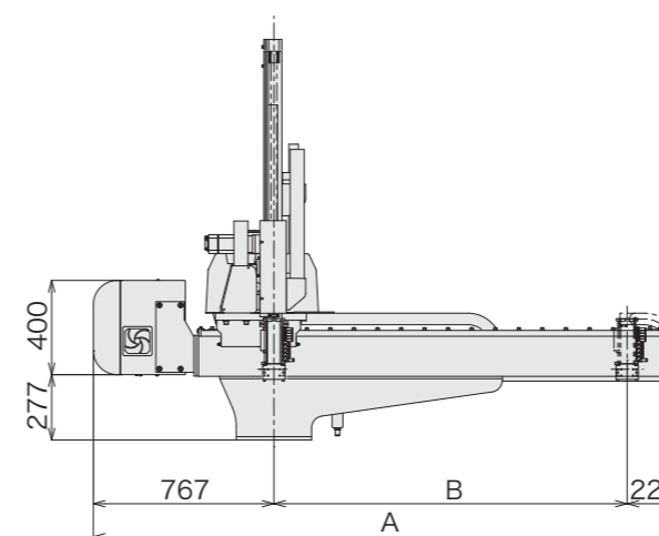
操作側取出仕様 (mm)
